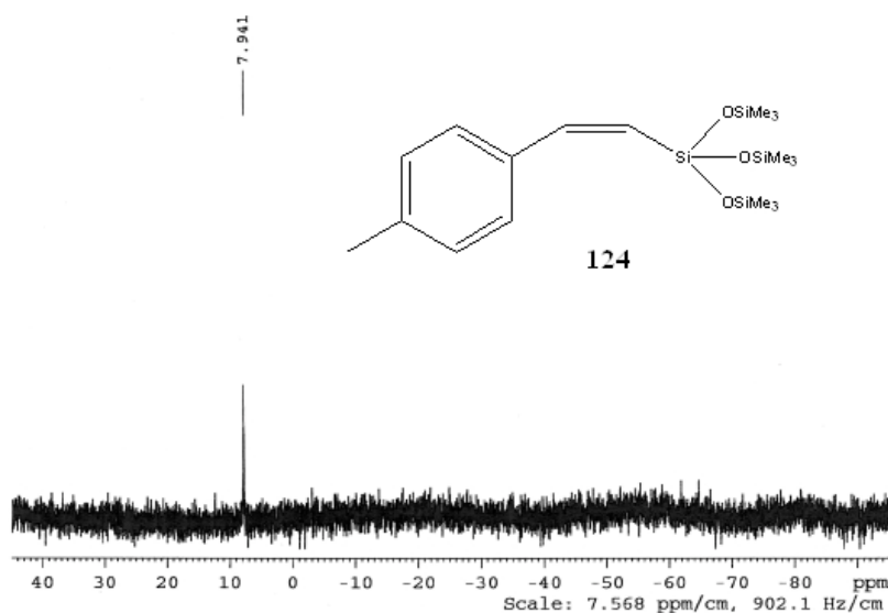
Figure 20. ^{29}\text{Si} NMR spectra of (Z)-2-(4-Methylphenyl)-1-[tris(trimethylsiloxy)silyl]ethane.
